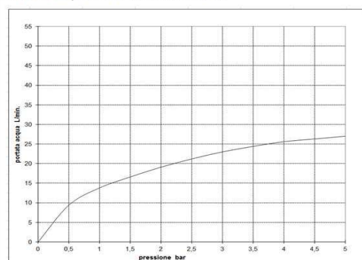
Grafico di portata / Flow rate diagram
